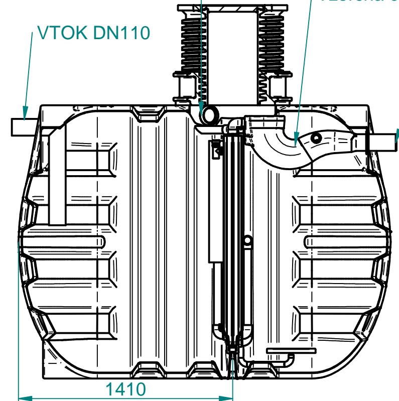
Section A-A
