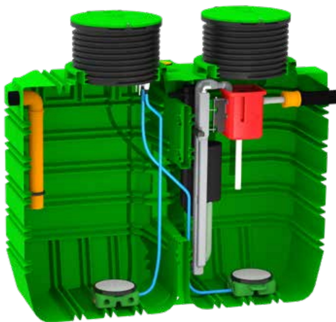
RoOxy 6 PU
