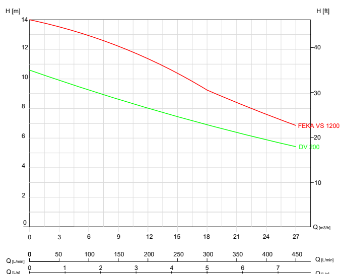
Pumpe FEKA VS 1200
